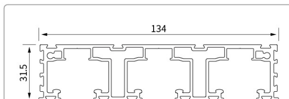
型号:YMHC19837J 名称:组合三吊轨
