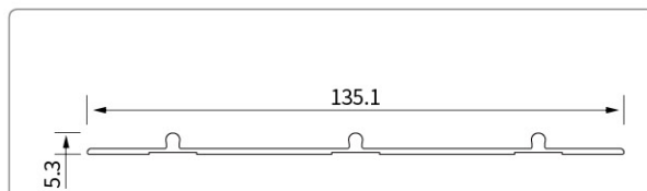
型号:YMHC19832 名称:三边封
