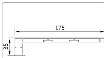
型号:YMHC17977 名称:175 连体系线
