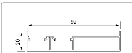
型号:YMHC19801 名称:组合双吊轨
