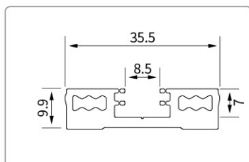
型号:YMHC19845 名称:特厚竖框
