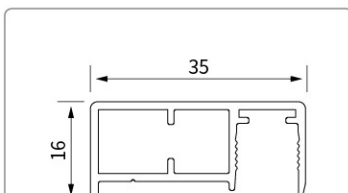
型号:YMHC18993 名称:35 门套
