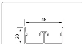
型号:YMHC19796 名称:组合单吊轨
