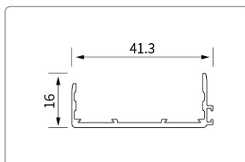
型号:YMHC19848 名称:勾企拍盖
