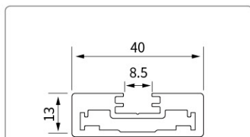
型号:YMHC19839 名称:特厚门框
