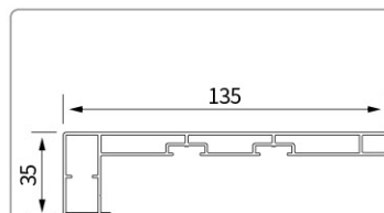
型号:YMHC17976 名称:135 连体系线
