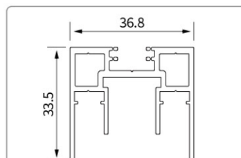
型号:YMHC19849 名称:上下横
