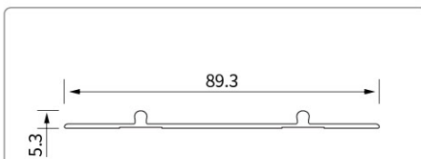
型号:YMHC19831 名称:双边封
