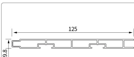
型号:YMHC17975 名称:连接板
