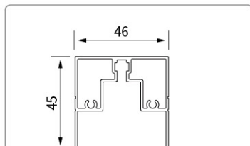
型号:YMHC19797 名称:单上轨
