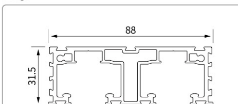
型号:YMHC19801 名称:组合双吊轨
