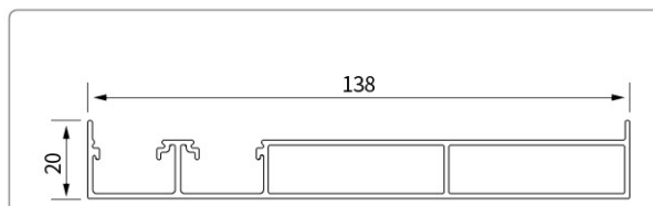
型号:YMHC19837J 名称:组合三吊轨
