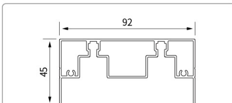
型号:YMHC19802 名称:双上轨
