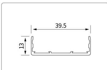
型号:YMHC19847 名称:光企拍盖
