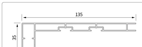
型号:YMHC17976 名称:135 连体套线
