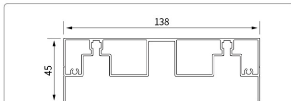
型号:YMHC19808 名称:三上轨
