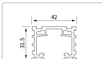
型号:YMHC19796 名称:组合单吊轨
