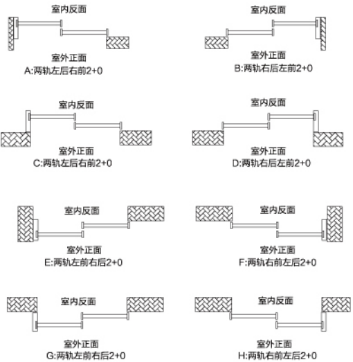
两轨2+0开启示意图
