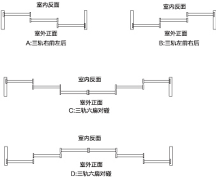
三联动开启示意图
