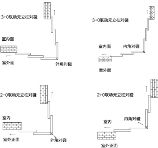
开放式无立柱对碰开启示意图
